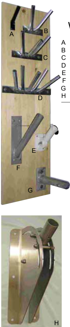
Wandhalter aus Stahl, 5fach, verzinkt, für Stäbe mit 15mmø
